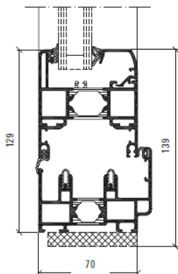
Vertikalsnitt ASS 70 FD
