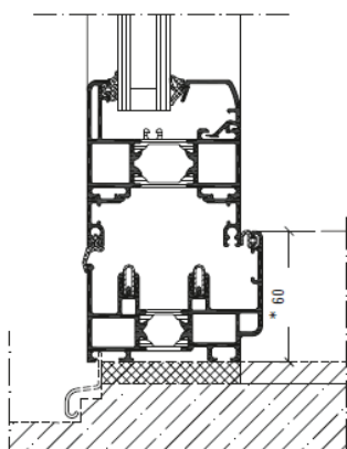
Tilslutningsprinsipp, foldesystem
