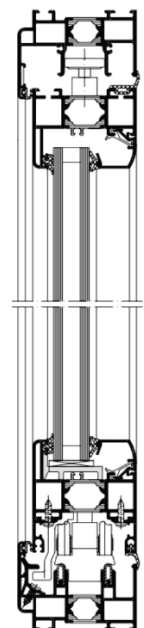
Horizontalsnitt av ASS 70 FD
